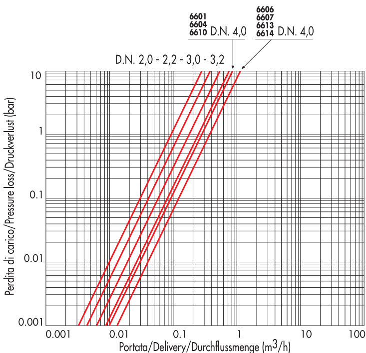
DIAGRAMMA PERDITA DI CARICO PRESSURE LOSS DIAGRAM
